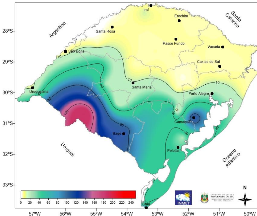
Chuva Ocorrida (mm) - 27/4/2018 a 03/5/2018
